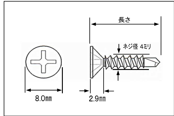
（皿 頭）
