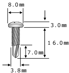
4×16
